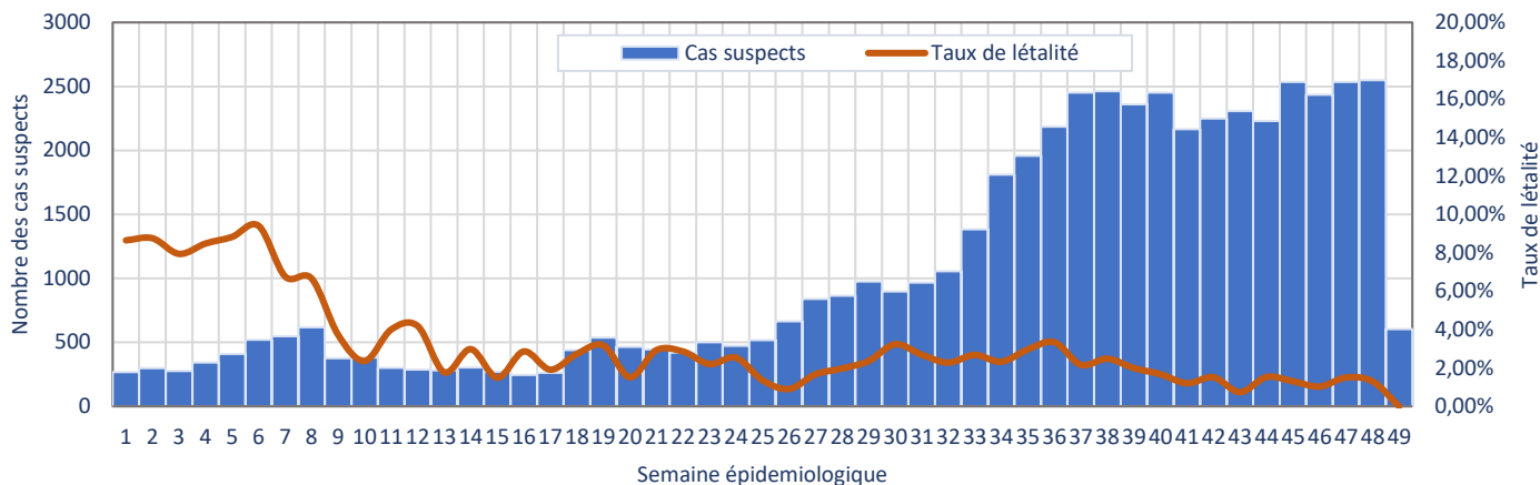
Figure 2. Courbe épidémique des cas et létalité suspects Mpox en RDC, S1-S49 - 2024
