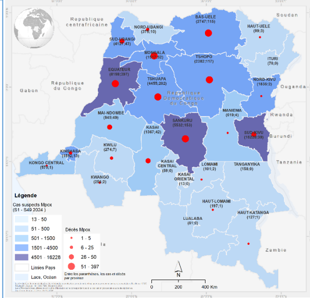
Figure 1. Répartition spatiale des cas suspects et décès de Mpx en RDC, S1-S50 2024
